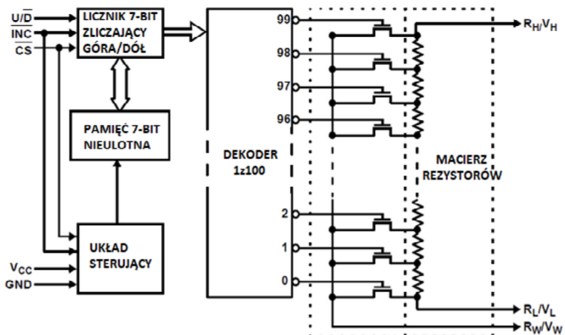
Przykład realizacji potencjometru cyfrowego
