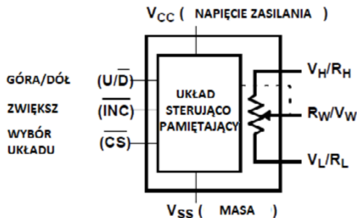
Potencjometr cyfrowy
